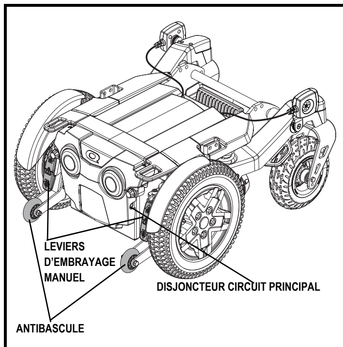
Figure 6. Base motorisée du Rival
