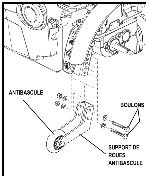
Figure 15. Roues antibascule
