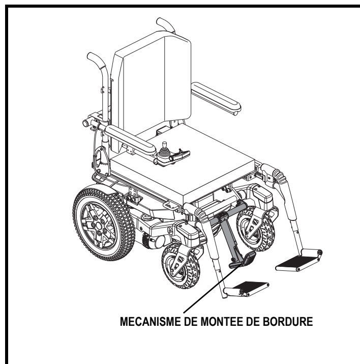
Figure 6A. Rival mécanisme de montée des bordures
